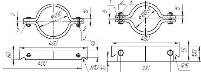
Хомут №1 1 – Скоба; 2 – Гайка М 16; 3 – Болт М 16х40; 4 – Болт М16х70 Хомут №2 Рисунок 3. Монтажные хомуты.
