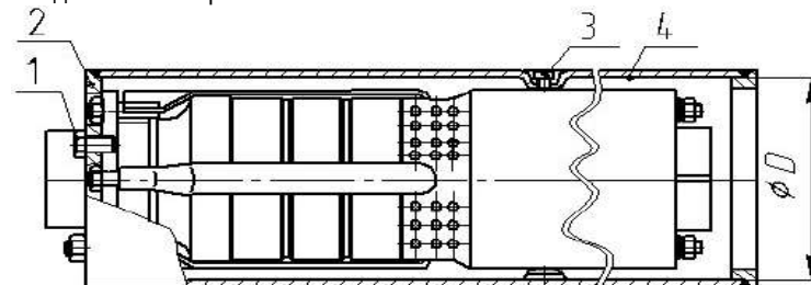
1 – Болт крепежный – 4шт. 3 – Центровочный винт 2 – Фланец кожуха 4 – Кожух
